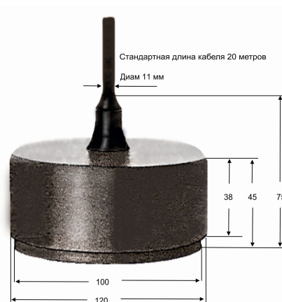
Антенна гидроакустическая TGM80-200
