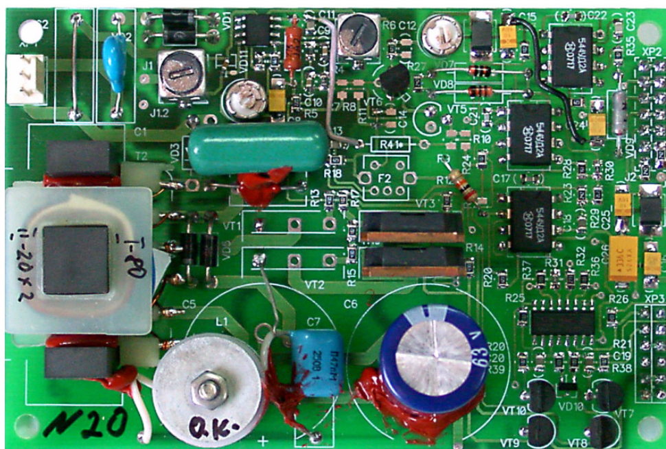
Внешний вид модуля TRX-1000--SI-12-50 кГц
