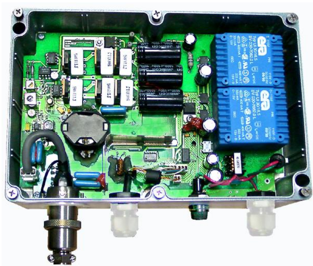
Бустер BU-4000 со снятой крышкой
